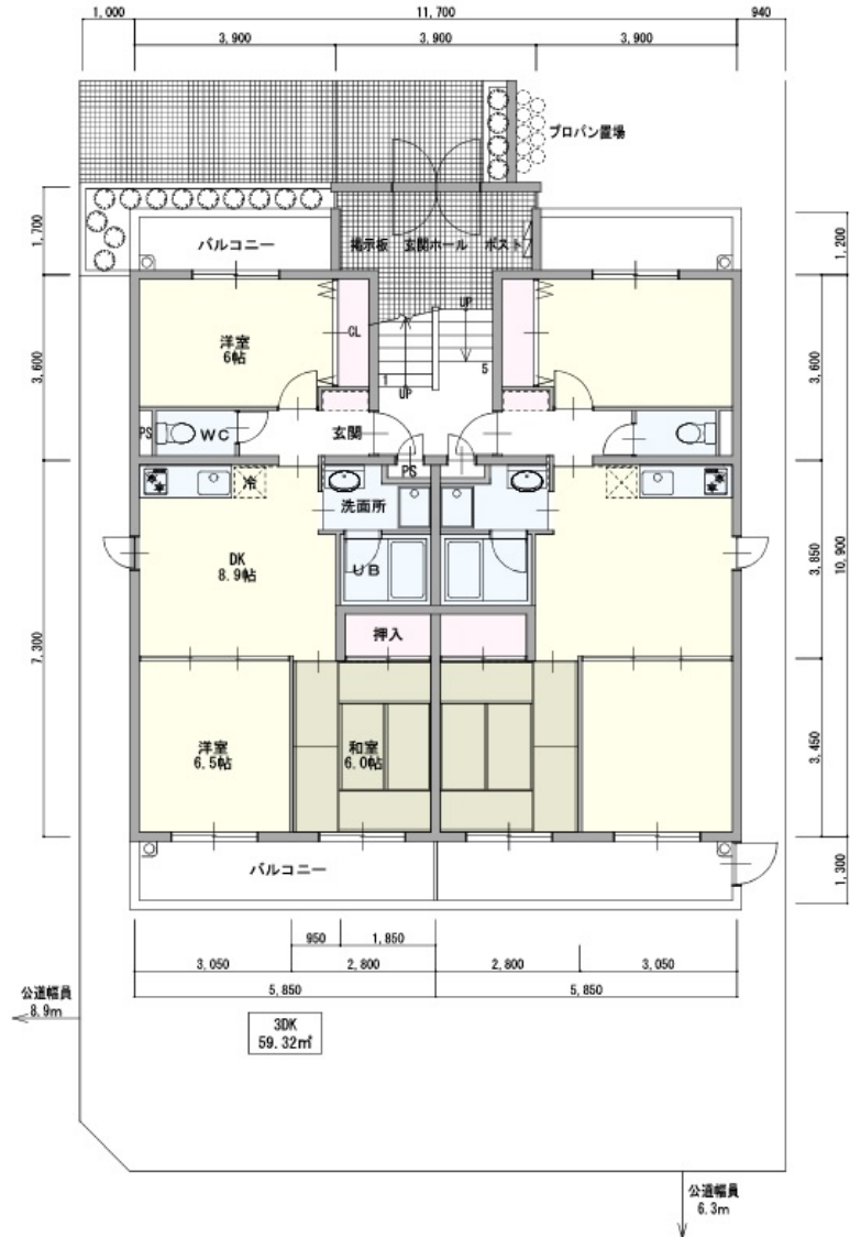
1F 平面図 1:100
